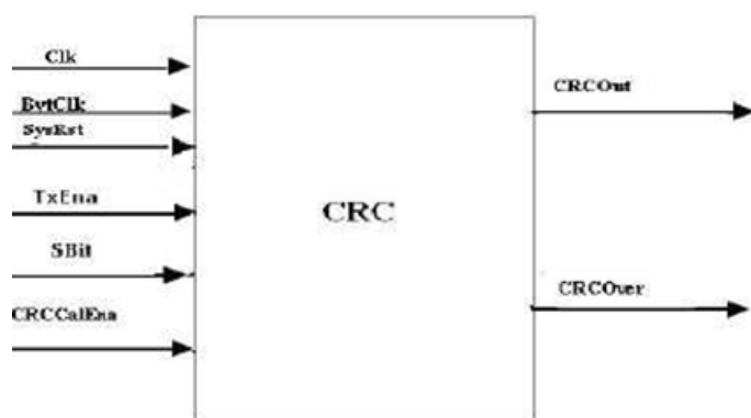
Fig 4.2c: CRC Module
