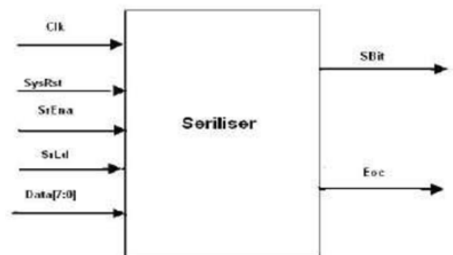
Fig.4.2(a): SerialiZer Module
