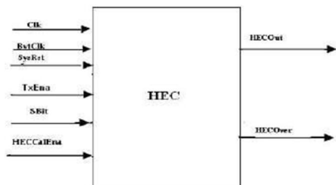
Fig 4.2b: HEC Module
