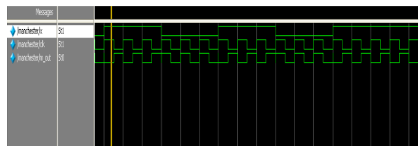
Manchester Coding
