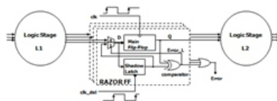
Fig: Razor flip flops.
