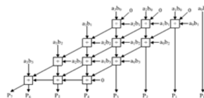
Fig: 4 \times 4 normal AM
