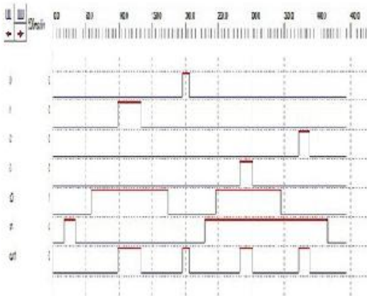
Fig.4- 4:1 MUX output
