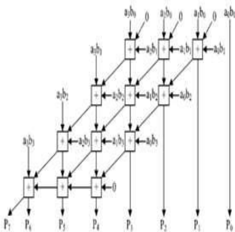
Fig. 1. 4 × 4 normal AM
