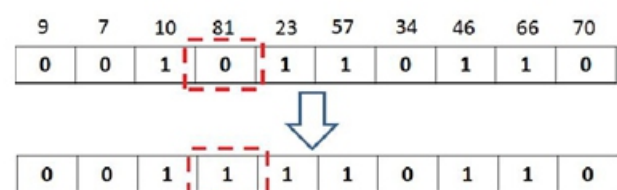
Fig. 7. Mutation step.
