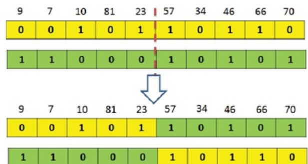
Fig. 6. Crossover step.
