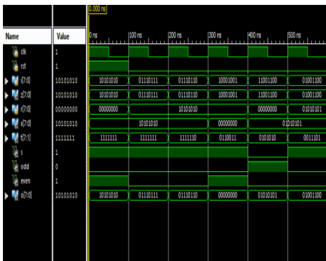
Fig.12. Scheme III Decoder.
