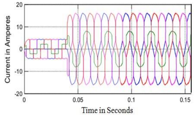
Fig 9. Source Current Due To Non Linear Load
