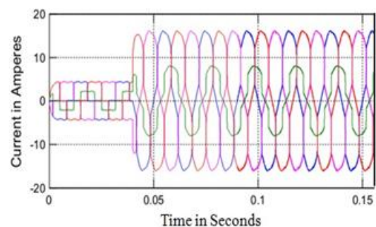
Fig 9. Source Current Due To Non Linear Load
