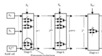
Fig. 3. n-input LUT
