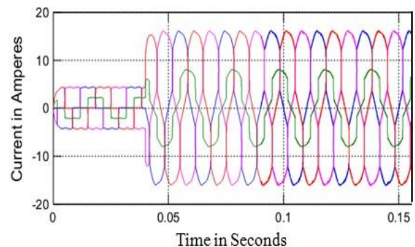
Fig.10: Source Current Due To Non Linear Load
