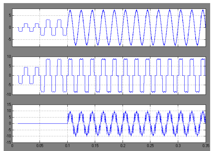
Fig.9: Compensation for non linear load
